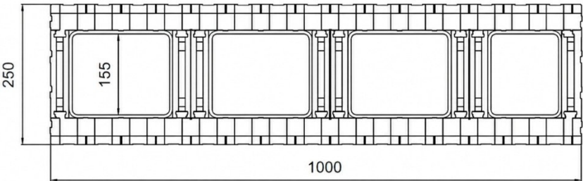
VISTA SUPERIOR
