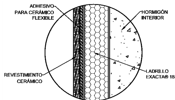
Revestimiento cerámico
