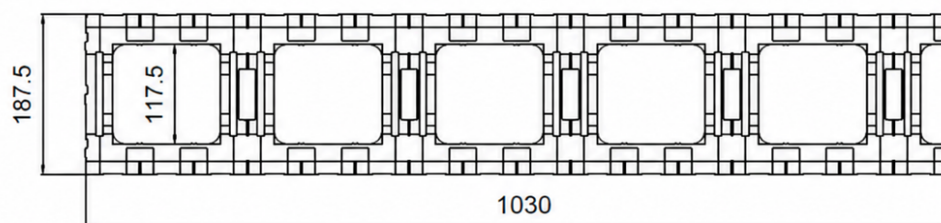
VISTA SUPERIOR
