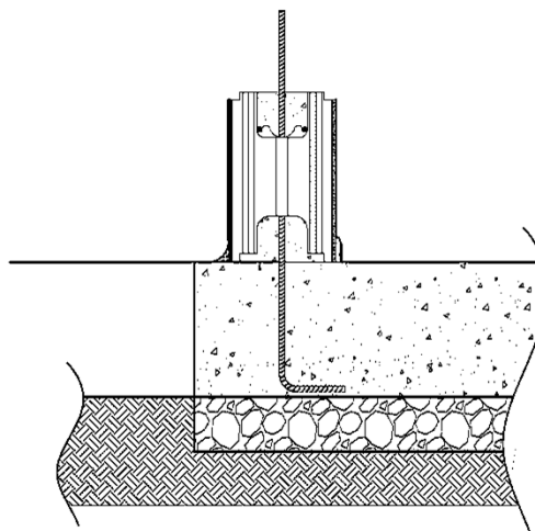
Anclaje de tensor a fundación
