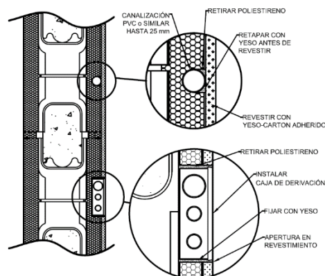
Instalaciones eléctricas
