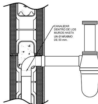
Instalaciones Sanitarias
