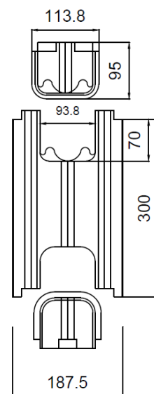
VISTA FRONTAL Y TAPAS
