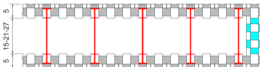
VISTA SUPERIOR
